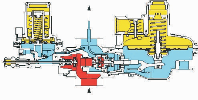
TYP CSB 404
