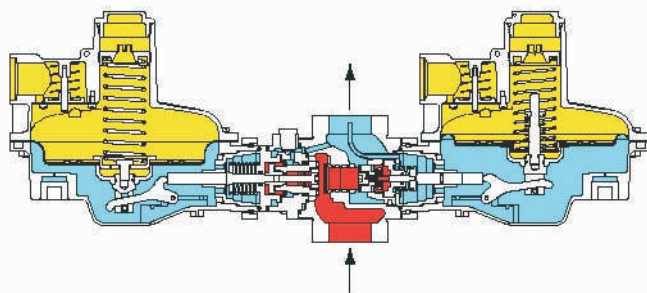
TYP CSB 403
